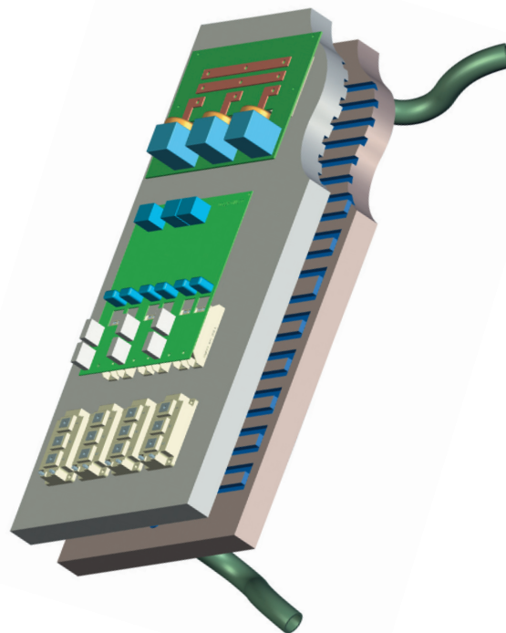
Refrigeración Fluid-Cooling
